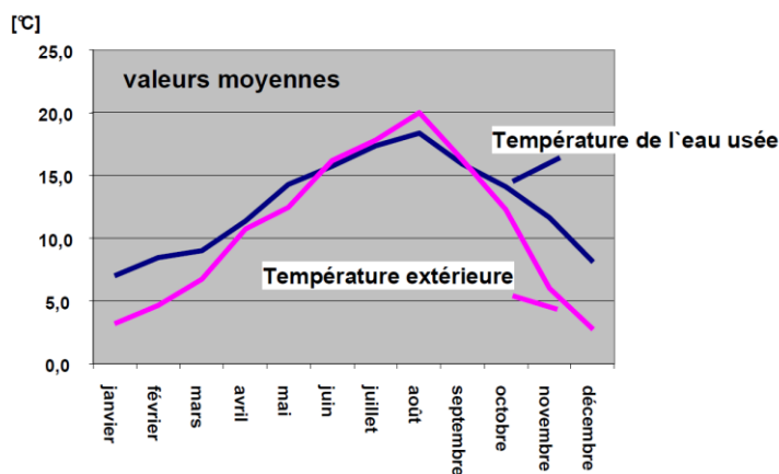
Evolution statistique moyenne des températures mensuelles
